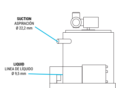
LEFT SIDE VIEW VISTA LATERAL IZQUIERDA
