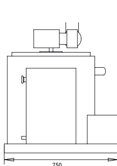
RIGHT SIDE VIEW VISTA LATERAL DERECHA
