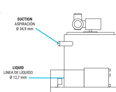
LEFT SIDE VIEW VISTA LATERAL IZQUIERDA
