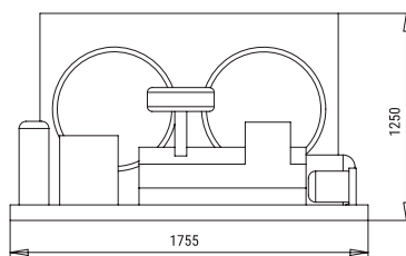
RIGHT SIDE VIEW VISTA LATERAL DERECHA
